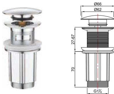
CP Plastic Pop up
