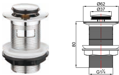
CP Plastic Pop up
