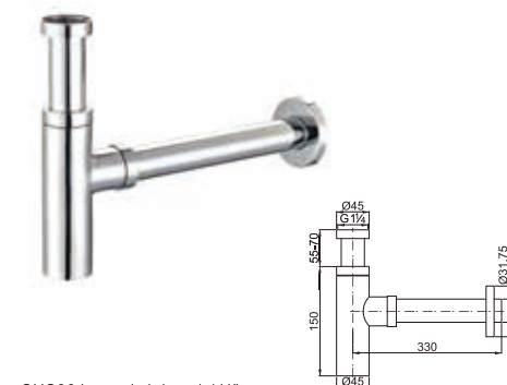
SUS304 round siphon 1 1/4"
