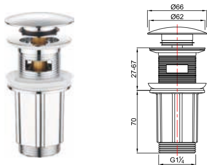
CP Plastic Pop up
