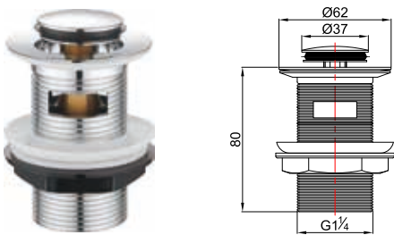
CP Plastic Pop up
